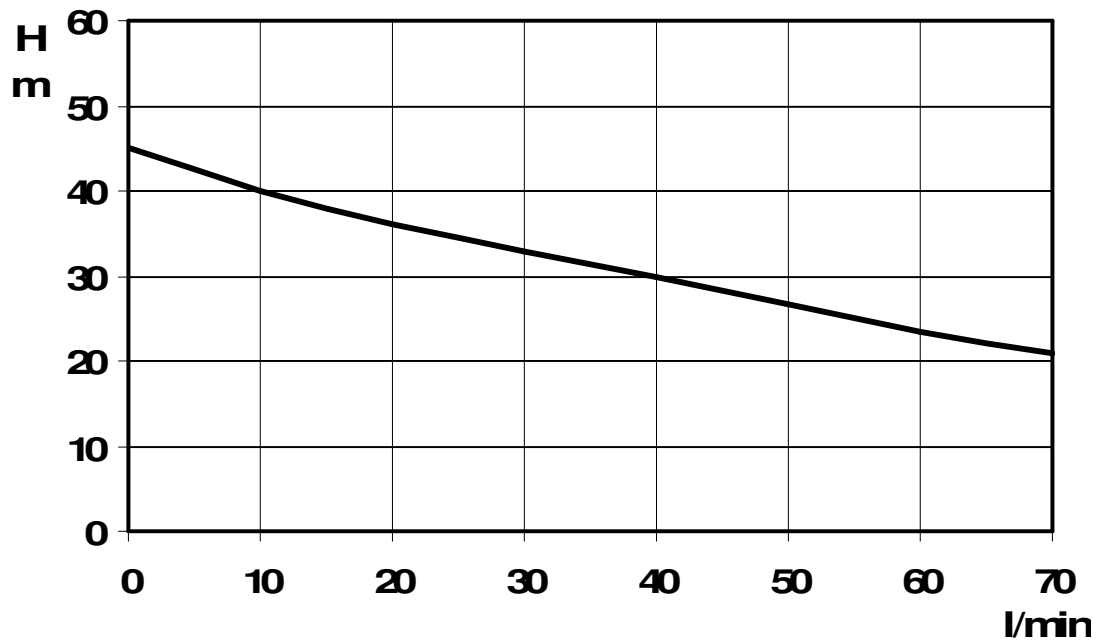
Kapacitetskurva
