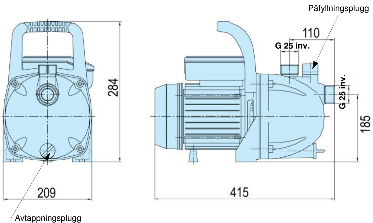
Måttskiss
